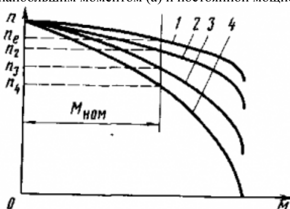
Рисунок 2 – Механические характеристики двухскоростных асинхронных двигателей с постоянным наибольшим моментом (а) и постоянной мощностью (б)
