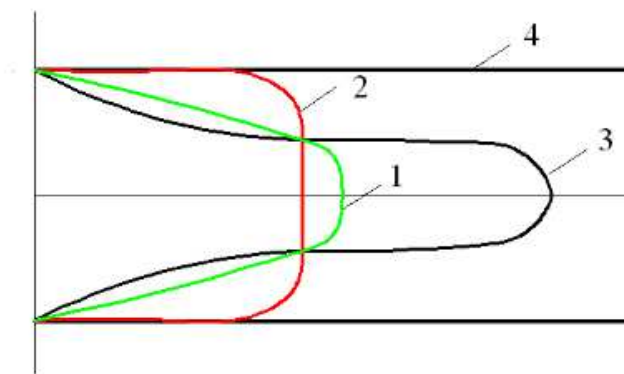
1 сурет – Мұнай температурасының оның құбырдағы ағын жылдамдығының таралуына әсері: 1 – мұнайдың изотермиялық ағыны; 2 – тұтқыр мұнайдың қыздырылуы; 3 – тұтқыр мұнайдың салқындауы; 4 – құбыр қабырғасы
