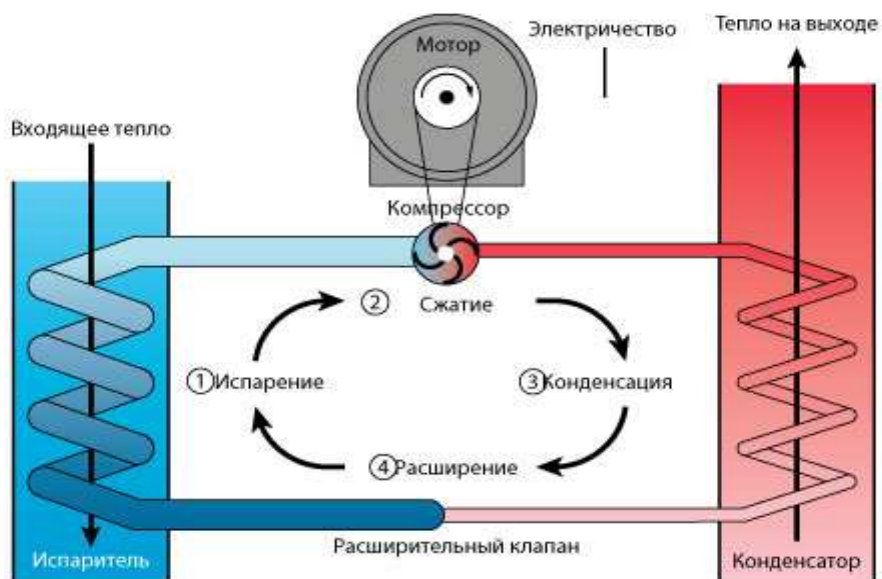
Рисунок 1 – Компрессионный тепловой насос
