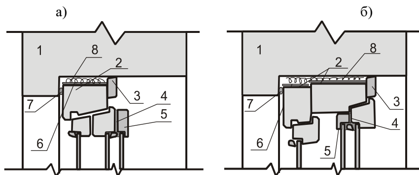
2 сурет – Алмалы салмалы өрімдер орнатылған өрімделген (а) және бөлек (б): 1 – қабырға; 2 – терезе қорабы; 3 – ішкі бөлініс; 4 – герметикалық төсеме; 5 – қосымша түптеу; 6 – рубероид; 7 – герметик; 8 – желдетпе.
