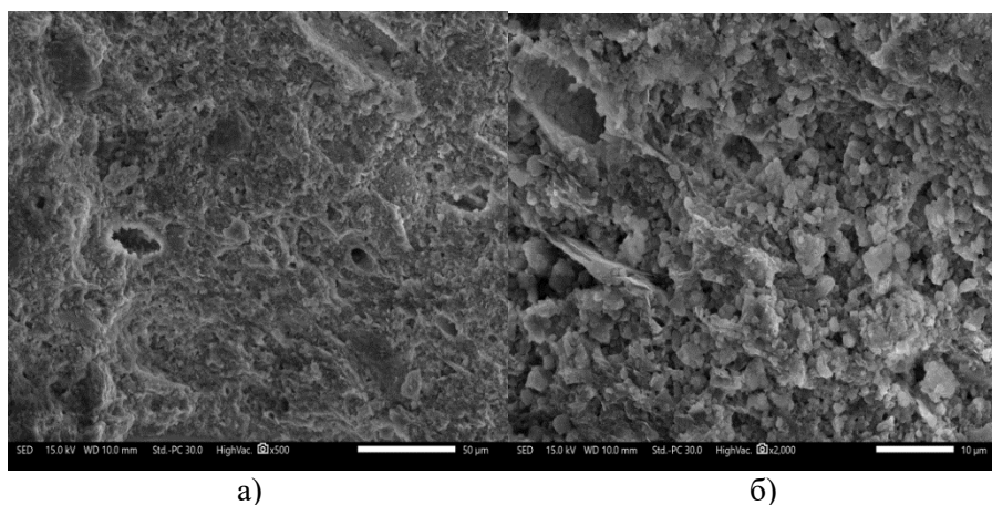
Рисунок 1 - Пористая структура кремнистой породы – опоки Таскалинского месторождения: а – увеличение \times 500 , б – увеличение \times 2000 (сканирующий электронный микроскоп JSM – IT 200)
