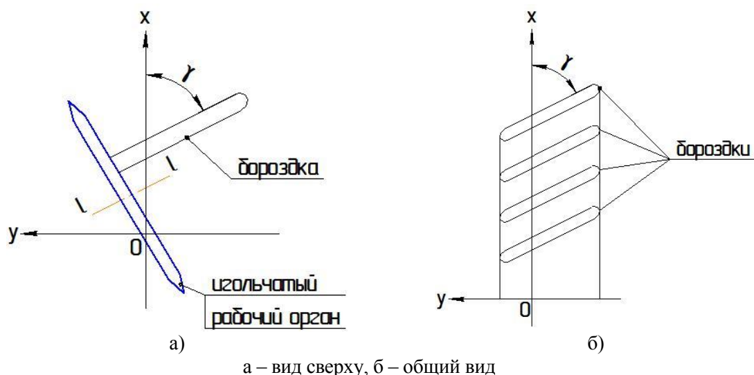
Рисунок 4 – Бороздообразование игльчатым рабочим органом
