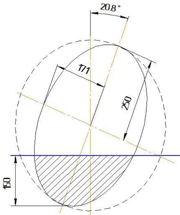
Рисунок 3 – Профиль дна борозды, формируемый дисковым рабочим органом
