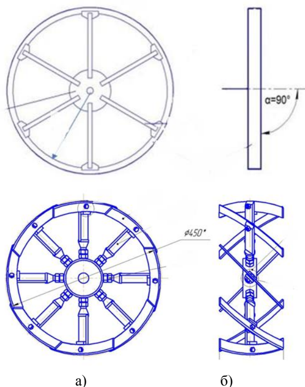
а – кольцевой рабочий орган; б – ножевой рабочий орган
