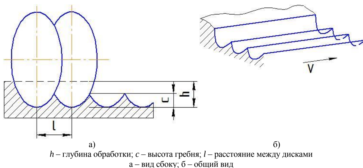
Рисунок 2 – Бороздообразование дисковыми рабочими органами
