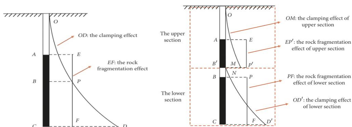
Рисунок 3 – Кривые эффекта зажима и эффекта фрагментации породы в зависимости от глубины. (а) Одноэтапная взрывная обработка. (б) Двухэтапная взрывная обработка. ((а) и (б) показаны различия между одноступенчатой и двухступенчатой струйной обработкой).
