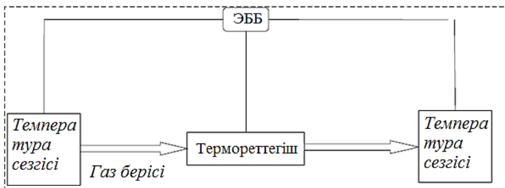
Сурет 3 – Отынды термореттеудің принципіалды сұлбасы
