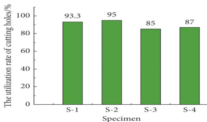
Рисунок 13 – Коэффициент использования вырубаемых скважин
