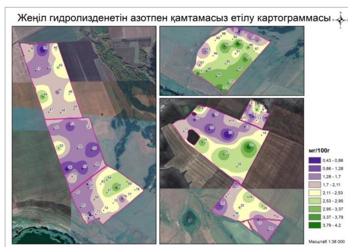
Сурет 4 – Қызығушылық аймағындағы топырақтағы азотты бағалауға арналған интерполяциялық модельдер
