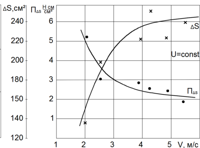
Рисунок 9 – Зависимость удельной поверхностной энергоемкости \Pi_{уд} и образованной поверхности образца \Delta S от скорости воздействия ударника
