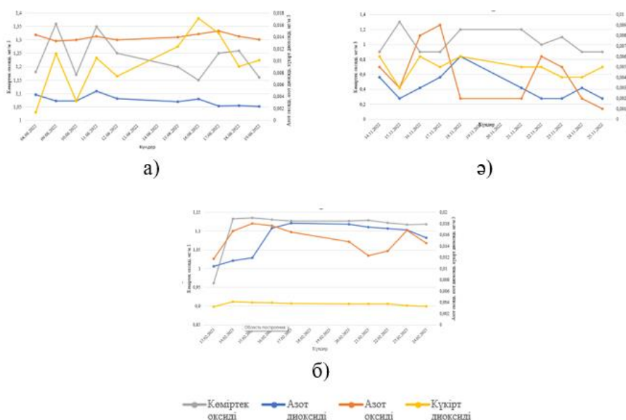
Сурет 1 – Негізгі ластаушы заттардың орташа күндік концентрациясы, \text{мг}/\text{м}^3 (а – 2022 жылдың тамыз айы, ә – 2022 жылдың қараша айы, б – 2023 жылдың ақпан айы)
