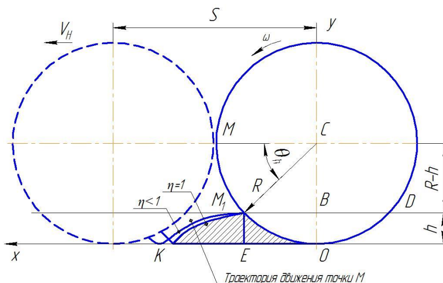
Рисунок 2 – Схема движения прикатывающего катка
