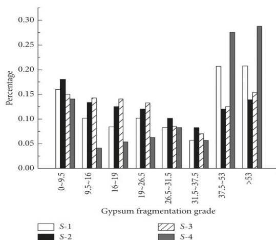
Рисунок 16 – Степень дробления при взрыве
