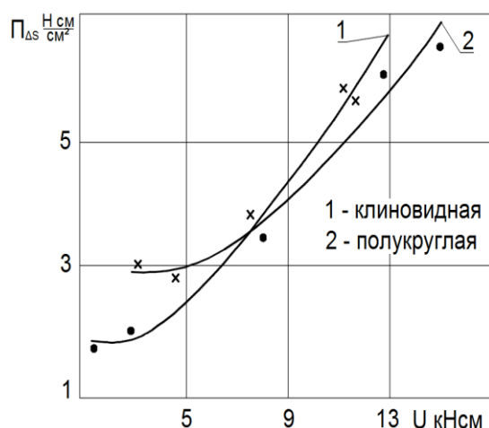
Рисунок 8 – Соотношение между удельной поверхностной энергоемкостью \Pi_{уд} и поглощенной энергией удара U для ударника с формой: 1.клиновидная; 2. полукруглая.
