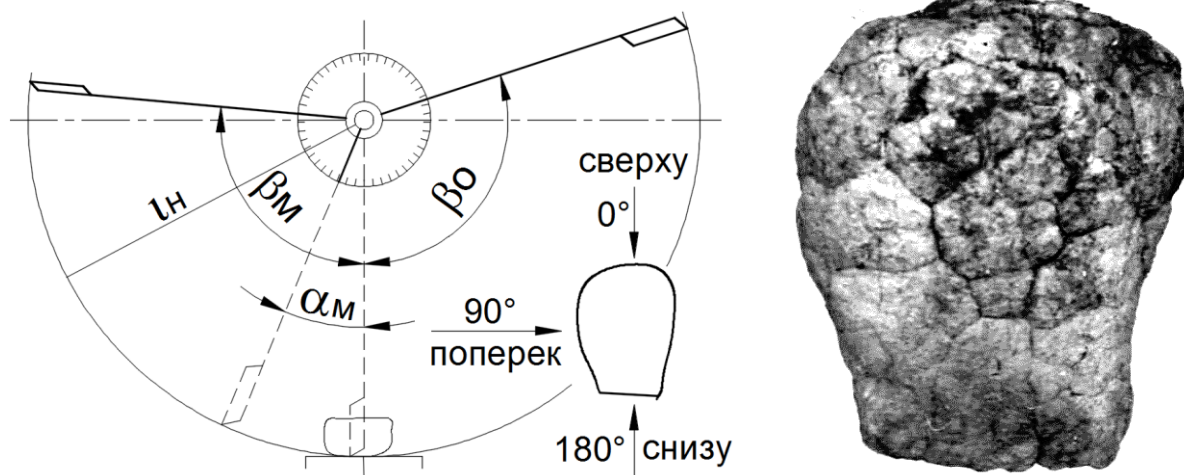
Рисунок 3 – Схема работы маятникового копра и столб солонца
