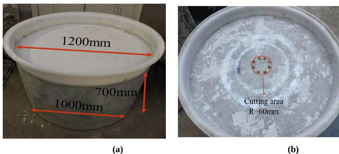
Рисунок 9 – Параметры образцов и площадь резания
