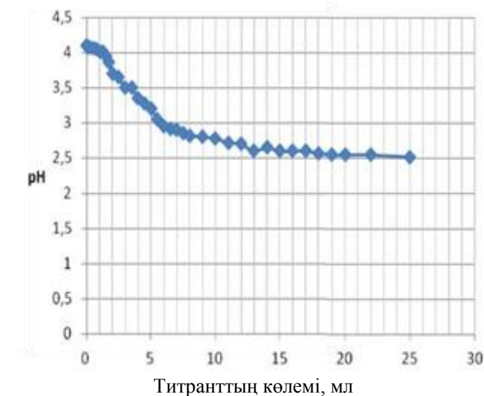
Сурет 2 – Титрант көлемінен ЛС-Na ерітіндісінің pH өзгеруі
