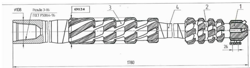
Рисунок 5 – Схема КФРГ-124.ИН
