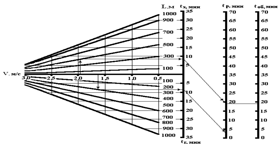
Сурет 3 - Тасымалдаушы көліктің айналым уақытын анықтауға арналған номограмма
