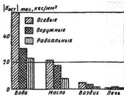
Рисунок 3 – Зависимость максимальных остаточных напряжений в цилиндрах (диаметр 50 мм) из углеродистой стали 0,3% С (закалка с 850°C, отпуск при 650°C) от охлаждающей среды
