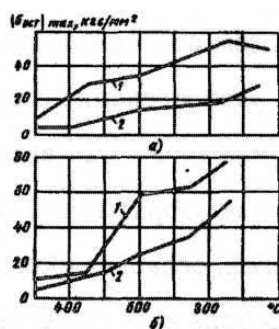
Рисунок 2 – Зависимость максимальных тепловых остаточных напряжений от начальной температуры.
