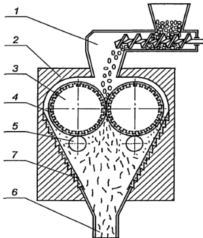
Рисунок 2 – Схемы вальцового станка: АС №882602
