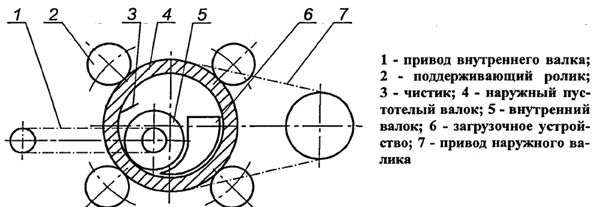
Рисунок 1 – Схема плющильной установки с внутренним контактом рабочих поверхностей
