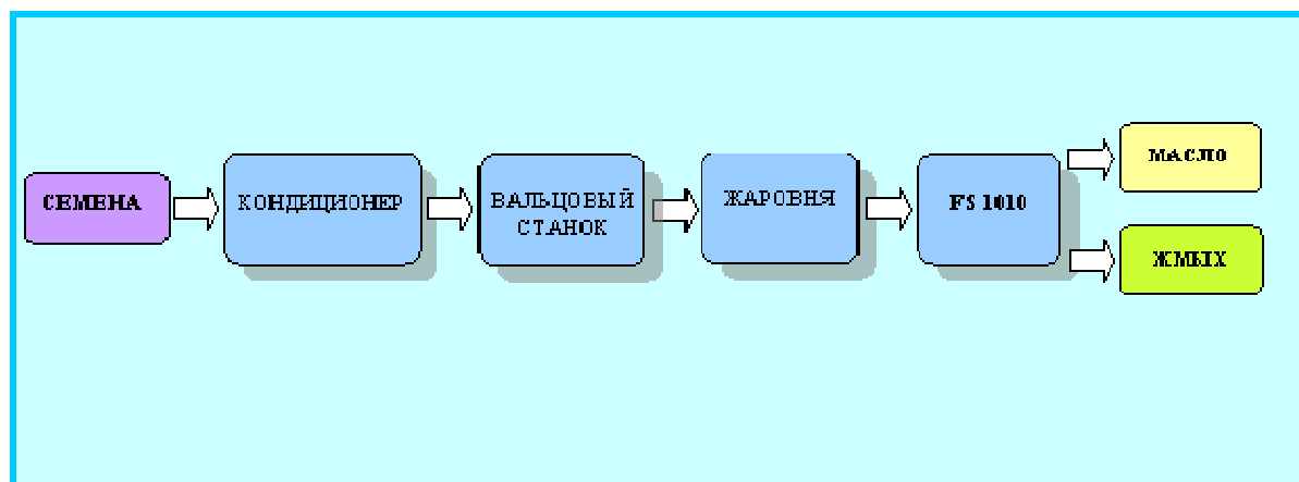
Рисунок 5 – Схема двукратного прессования горячим способом
