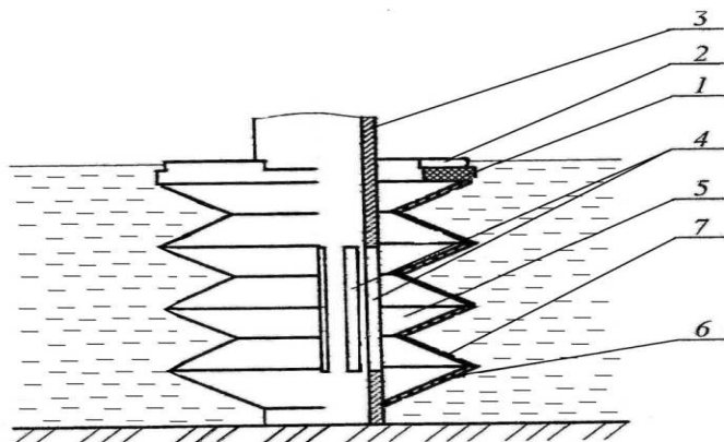
5 сурет – Батыс Қазақстан аграрлық-техникалық университетінде жасалған суды бетінен сорып алатын құрылғының конструктивтік – технологиялық сұлбасы
