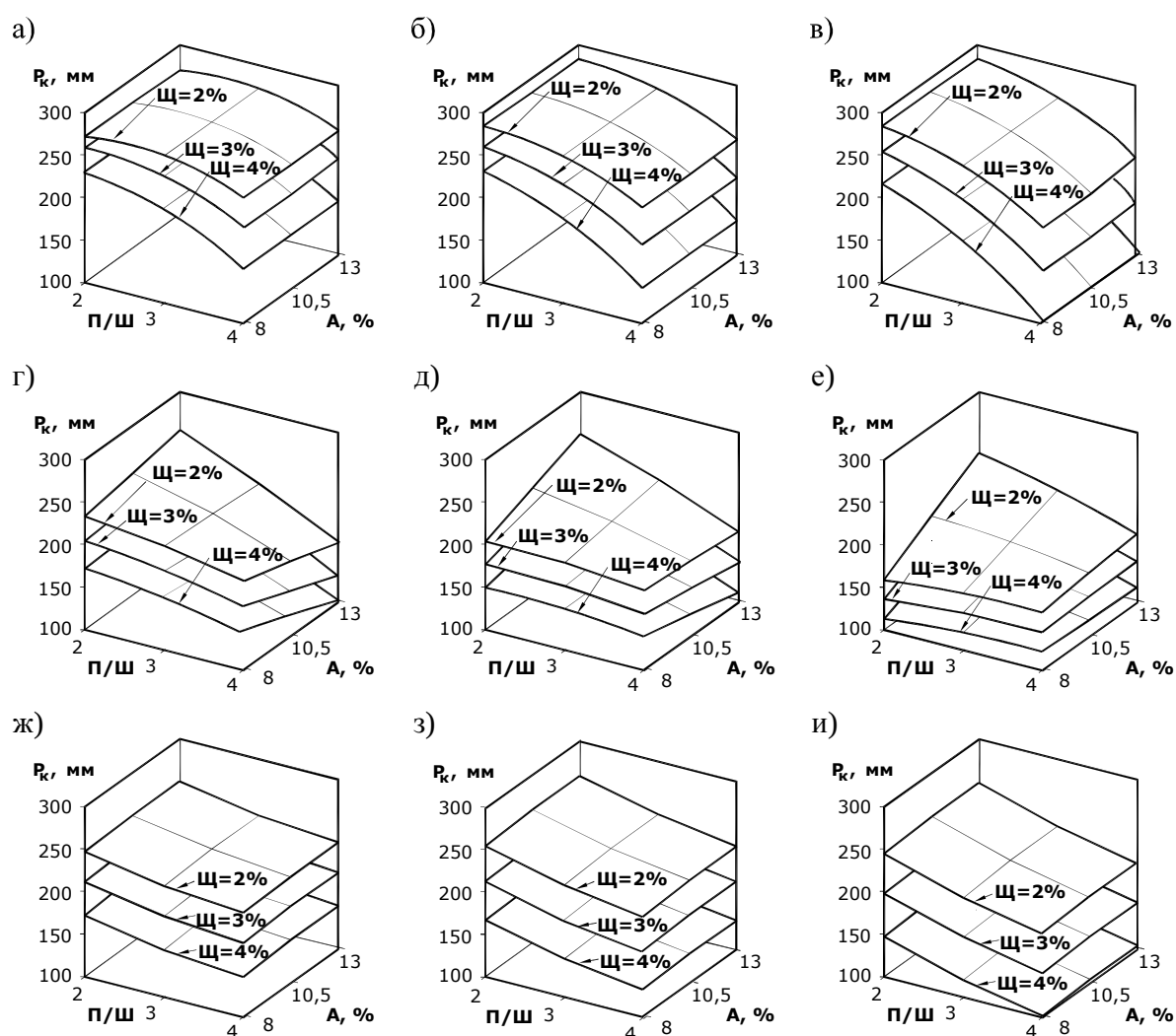
Рисунок 1 – Влияние соотношения горной породы и шлака в вяжущем П/Ш, расхода активатора А и щелочи Щ на расплывы растворных смесей, приготовленных на основе габбро-диабазы
