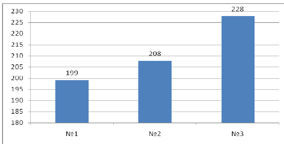
2 сурет – Рапс майының әртүрлі қоспасындағы Д-240 қозғалтқышының меншікті отын шығыны ( g_e , г/эф.а.к.с.).
