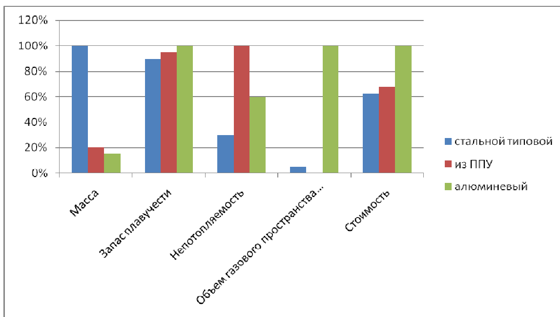
Рисунок 1 - Некоторые характеристики основных типов внутренних плавающих покрытий
