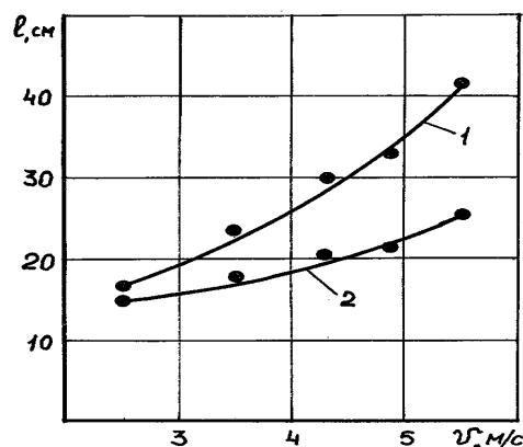
Рисунок 3 – Зависимость дальности полета отраженных зерен пшеницы от скорости падения при углах наклона отражателя: 1- \alpha = 30^\circ ; 2- \alpha = 40^\circ
