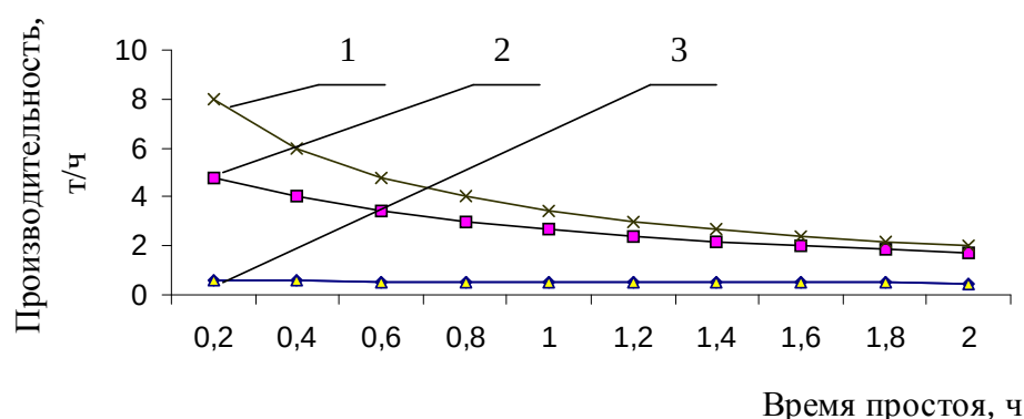
Рисунок 1 – Зависимость производительности автомобиля от времени простоя под погрузкой и разгрузкой при перевозках на расстояние: 1 – 5 км, 2 – 10 км, 3 – 100 км
