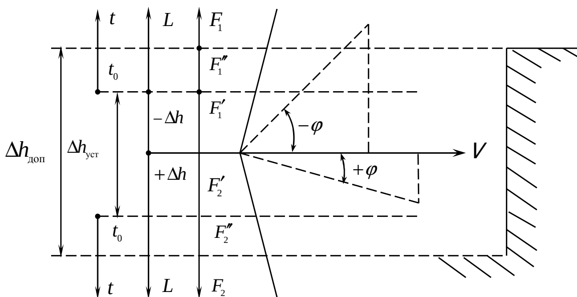
F_1, F_2 – частоты генераторов; -\Delta h, +\Delta h – отклонение по глубине; \Delta h_{уст} – установочное отклонение; L – линейное отклонение; t – временное отклонение; \Delta h_{доп} – допустимое отклонение
