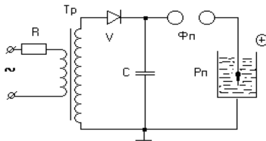
R – разрядное сопротивление, Tr – трансформатор, V – выпрямитель, ФП – формирующий промежуток, РП – рабочий искровой промежуток в жидкости, С – конденсаторная батарея
