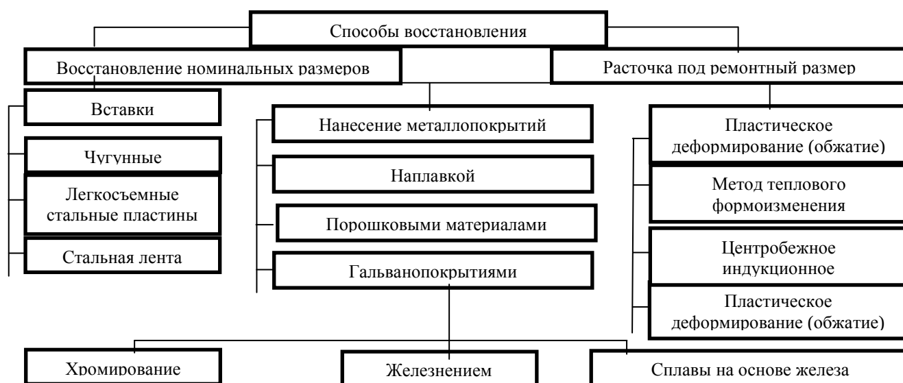
Рисунок 1 – Способы восстановления изношенных гильз цилиндров
