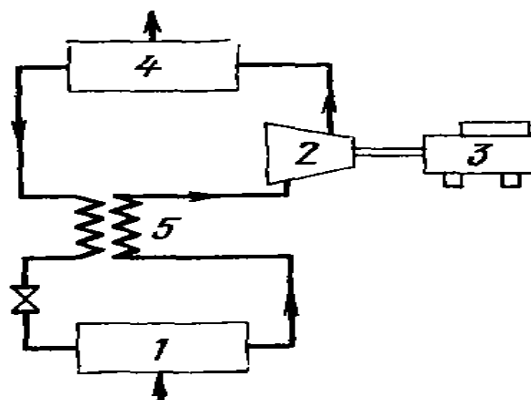
Рисунок 2 – Парокомпрессионный цикл с промежуточным теплообменником регенератором 1-испаритель; 2-компрессор; 3-двигатель; 4-конденсатор; 5-промежуточный теплообменник
