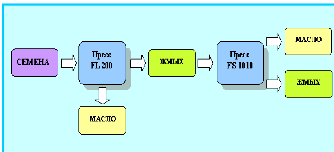
Рисунок 4 – Схема двукратного прессования холодным способом
