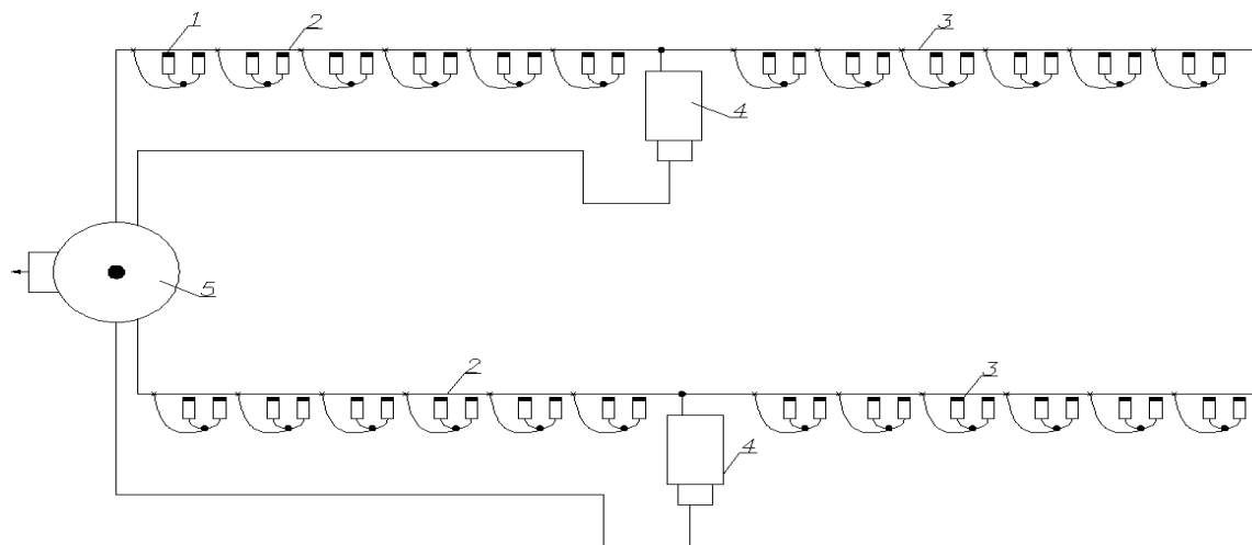
3 сурет – Стационарлы сауын қондырғыларының сүт өткізгіштерінің біріктірілуі
