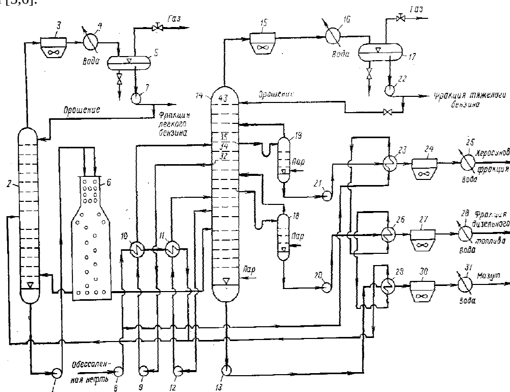
Рисунок 1 – Схема реконструкции установки атмосферной дистилляции нефти 1,7-9,12,13,20-22 – насосы; 2,14 – ректификационные колонны; 3,15,24,27,30 – аппараты АВО; 4,16,25,28,31 – холодильники; 10,11,23,26,29 – теплообменники; 5,17 – газосепараторы; 6 – трубчатый печь; 18,19 – отпарные колонны
