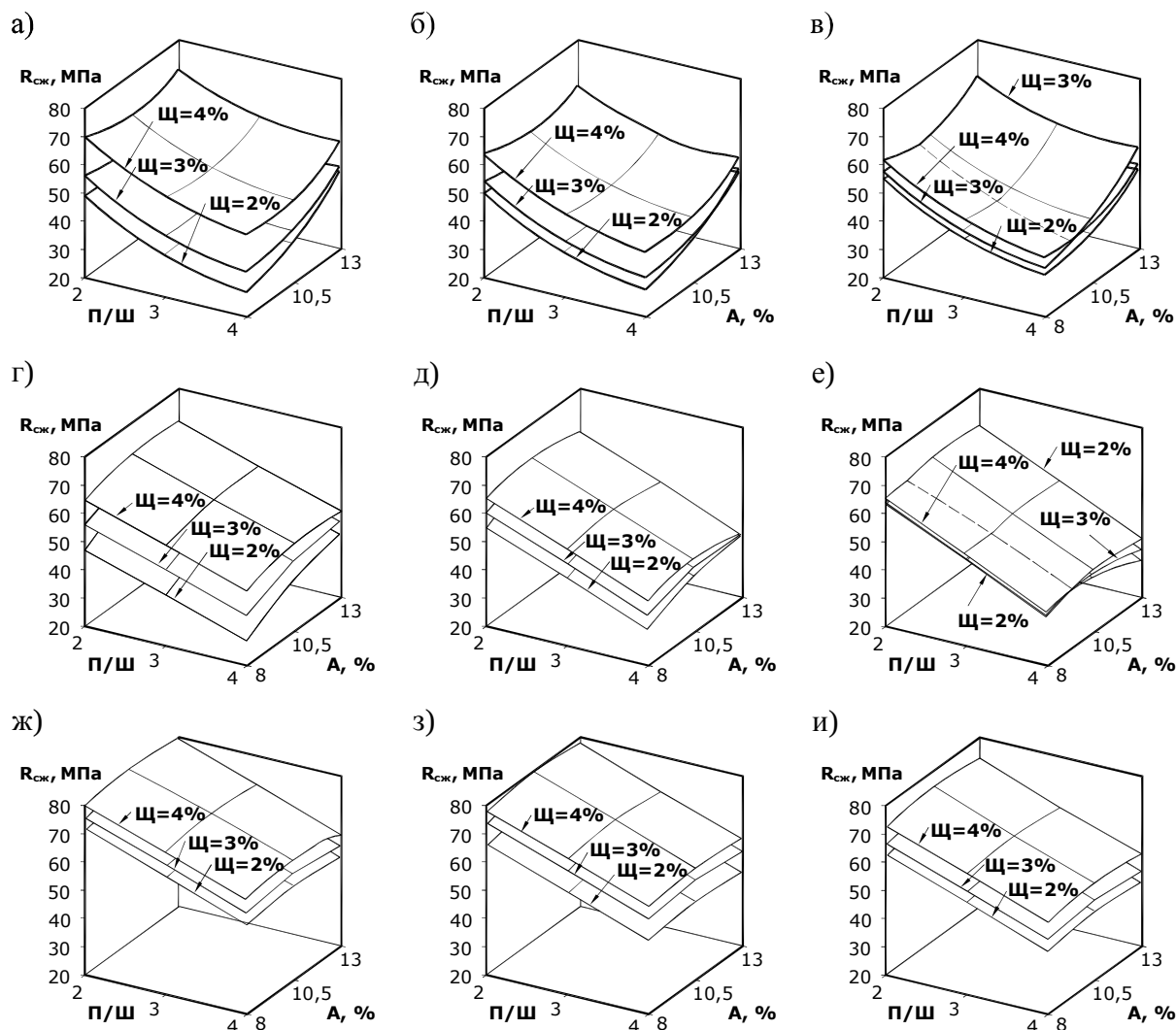
Рисунок 3 – Влияние состава минерально-щелочного вяжущего на прочность после тепловой обработки (обозначения по рис. 1)
