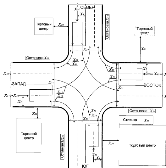
Рисунок 1 – Классификационные признаки регулируемых перекрестков
