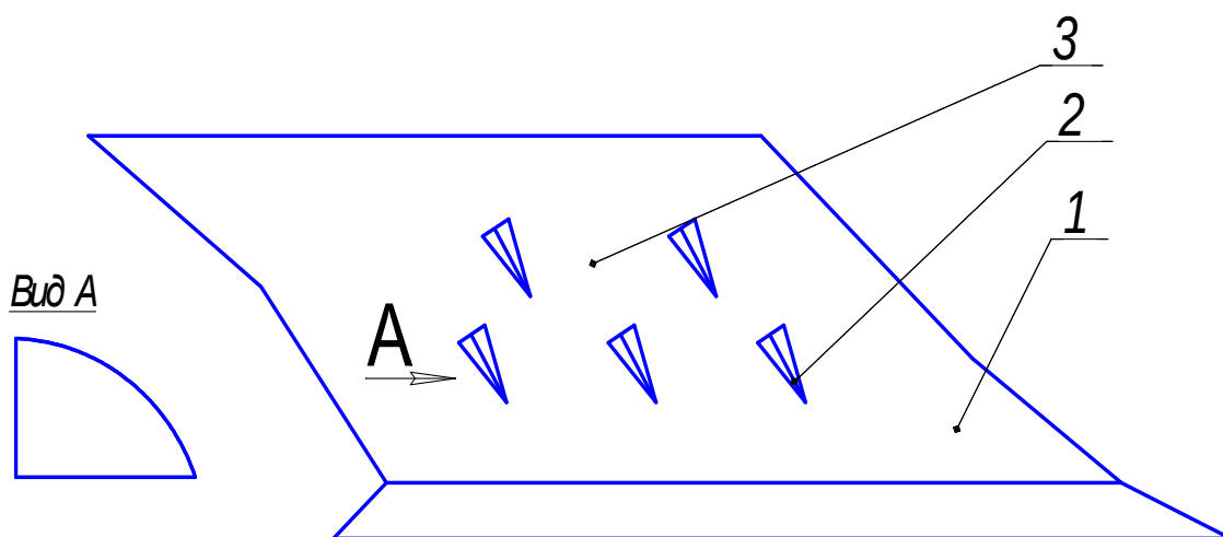
Рисунок1 – 1-Корпус плуга; 2- рыхлящие элементы; 3- грудь отвала.
