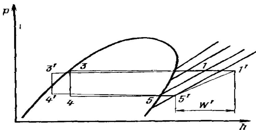
Рисунок 1 – Реальный парокомпрессионный цикл
