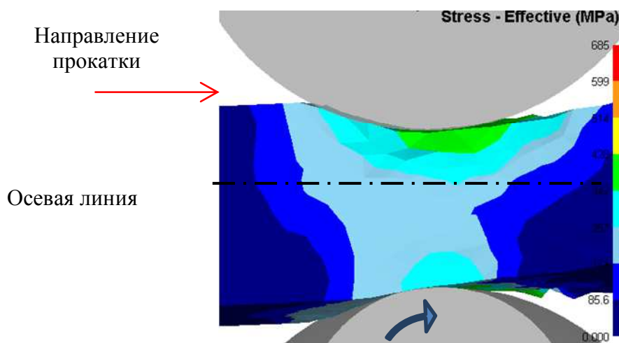
Рисунок 2 – Распределение эквивалентных напряжений по сечению полосы в процессе прокатки в валках с обратной конусностью
