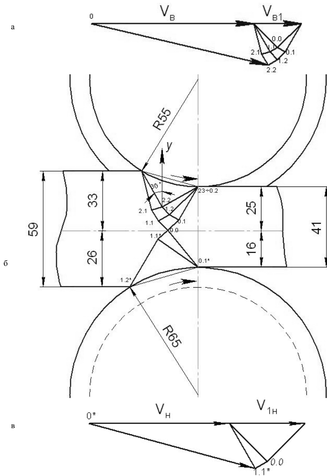
Рисунок 1– Поле линий скольжения (б) и поле скоростей со стороны верхнего (а) и нижнего валков (в)
