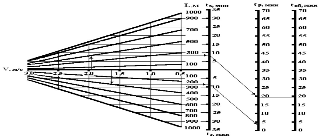
4 сурет – Тасымалдауыш көліктің айналым уақытын анықтауға арналған номограмма
