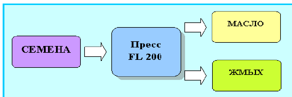
Рисунок 1 – Схема однократного прессования холодным способом
