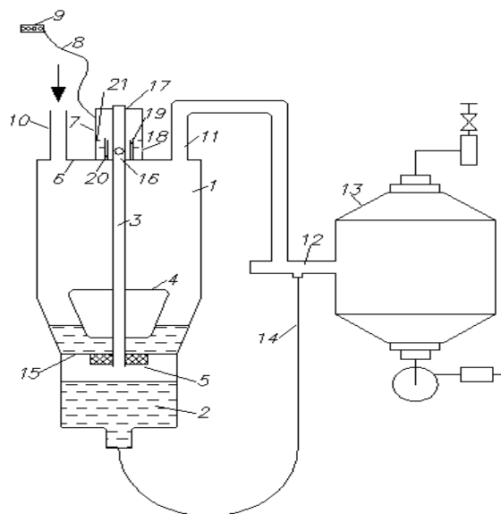
5 сурет – Сүтті есептеуіш-эвакуаторының сызбасы
