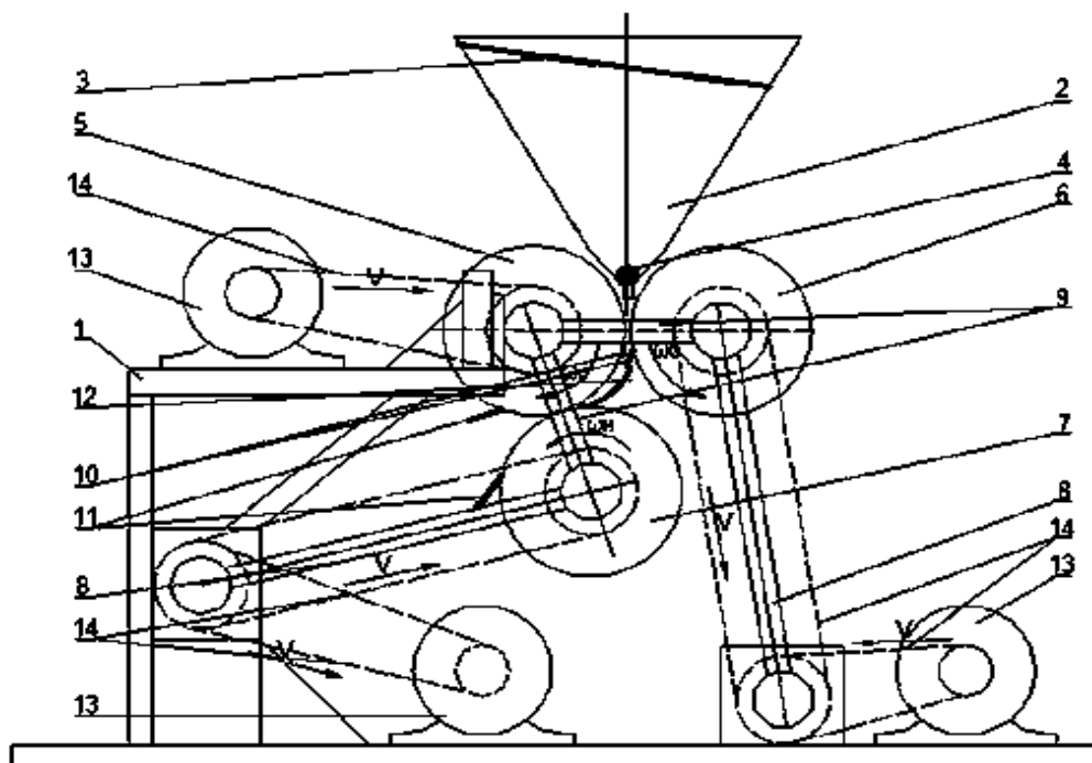
Рисунок 3 – Схема двухступенчатой плющилки зерна.
