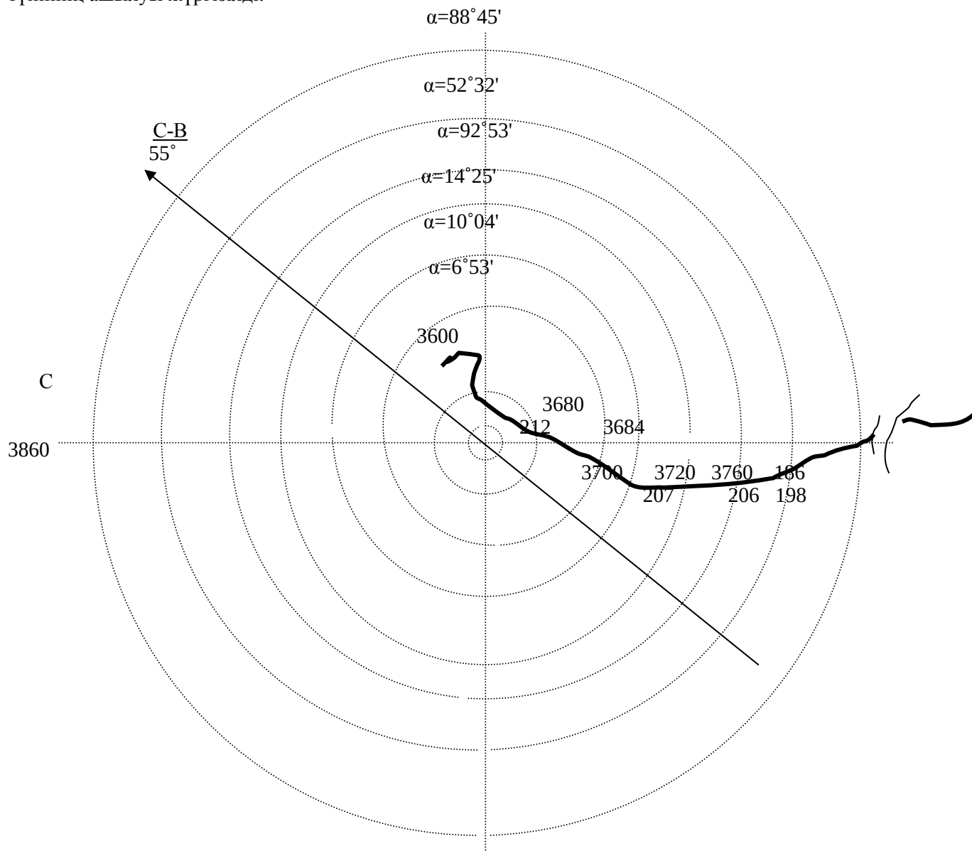
4 сурет-2407 ұңғыманың зениттік бұрышы мен азимуттың нақты пішіні
