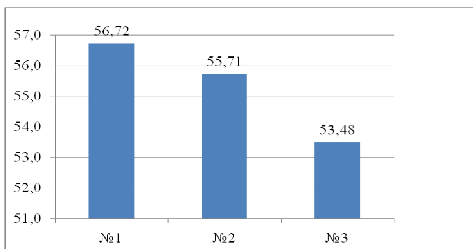
1 сурет – Өсімдік майының әртүрлі қоспа Д-240 қозғалтқышының тиімді қуаты ( N_e )
