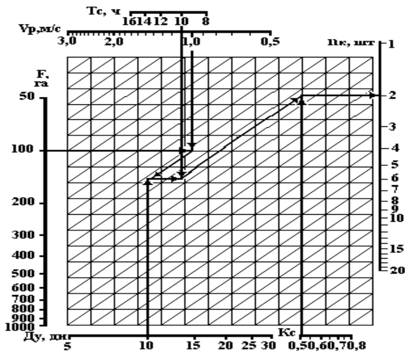
1 сурет – Қызылша қазғыштың мөлшерін анықтауға арналған номограмма
