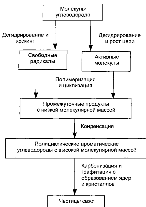
Рисунок 1 – Схема образования сажевых частиц
