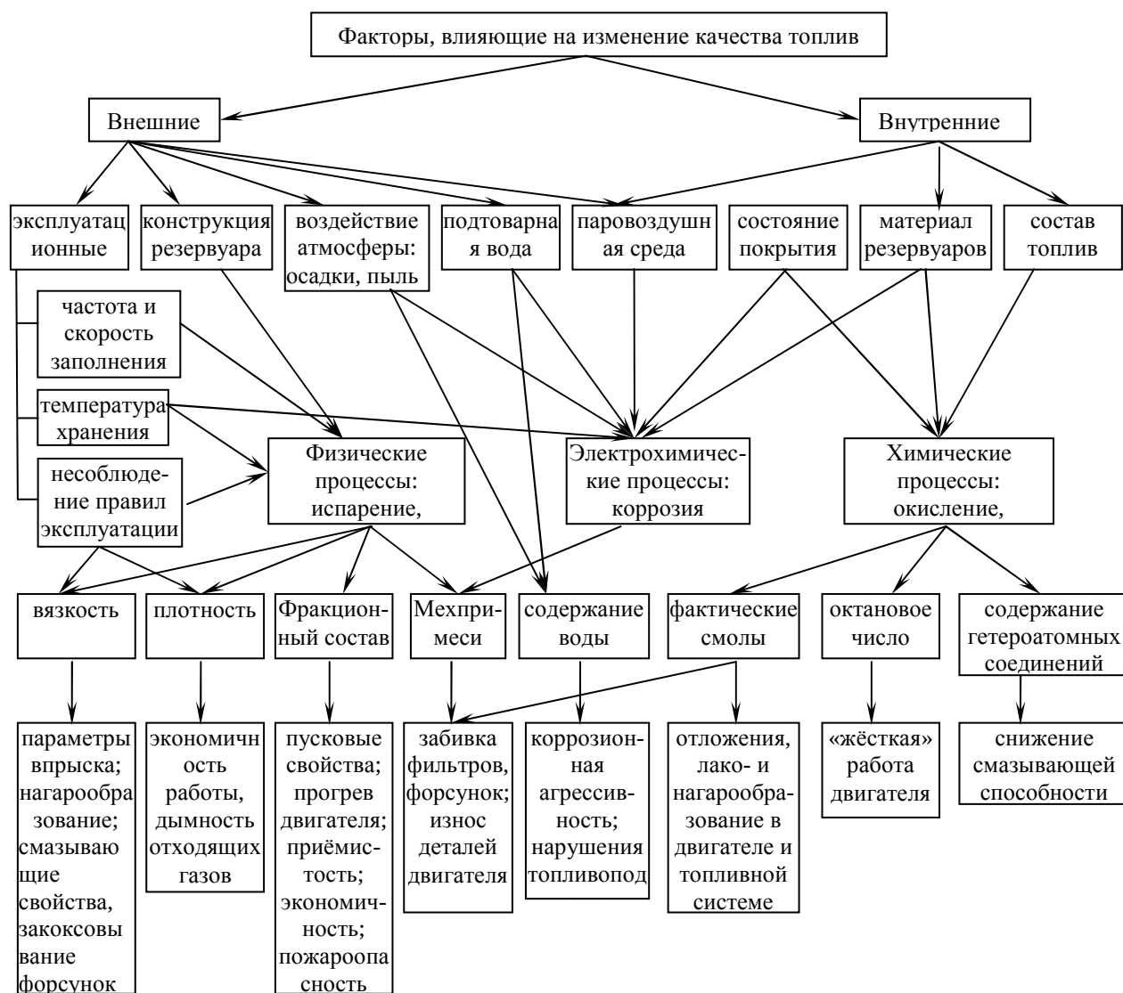
Рисунок 1 – Факторы, влияющие на снижение качества нефтепродуктов и работоспособность техники
