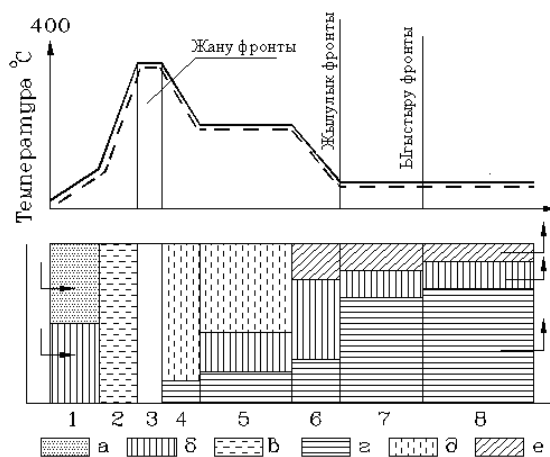
1 сурет – Ылғалды жандыру процесінің сұлбасы
