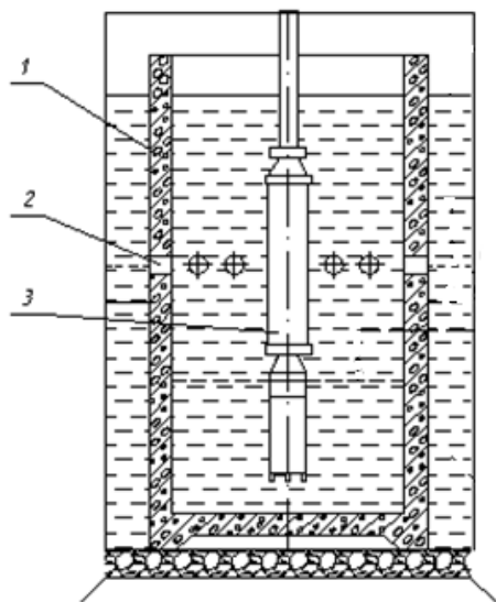
1 сурет – М. И. Калинин атындағы Түркімен ауыл шаруашылық институтында жасалған су айырғыш стакан конструкциясының сұлбасы 1 - корпус; 2 – тесіктер; 3 – сораптық агрегат
