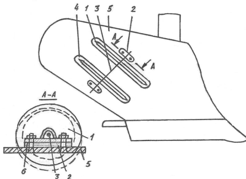
1 сурет – Соқа тұрқасы 1-қопсытқыш элементтер, 2-подшипник, 3-білік, 4-жырға, 5-қайырма, 6-төсем
