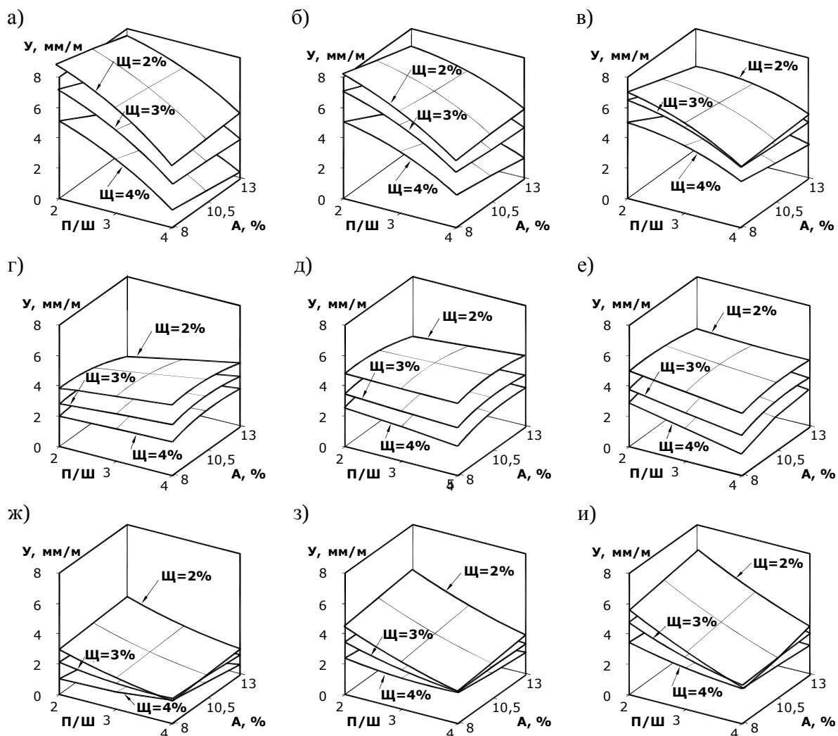
Рисунок 4 – Влияние состава минерально-щелочного вяжущего на усадку через 28 суток твердения в нормальных условиях (обозначения по рис. 1)
