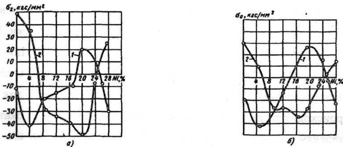
Рисунок 5 — Суммарные остаточные напряжения в зависимости от содержания Ni в стали с 0,03— 0,06% С. (Закалка с 900°С в воду при 0°С [11]):
