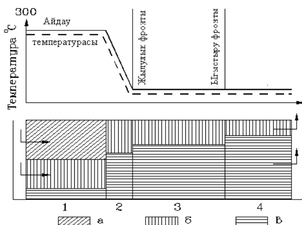
2 сурет – Мұнайды бумен ығыстырудың сұлбасы.
