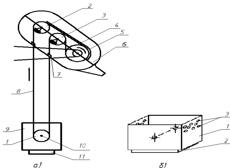
Сурет 2 – Батыс Қазақстан ауыл шаруашылық институтында жасалған лайлануға қарсы құндақ конструкциясының сұлбасы
