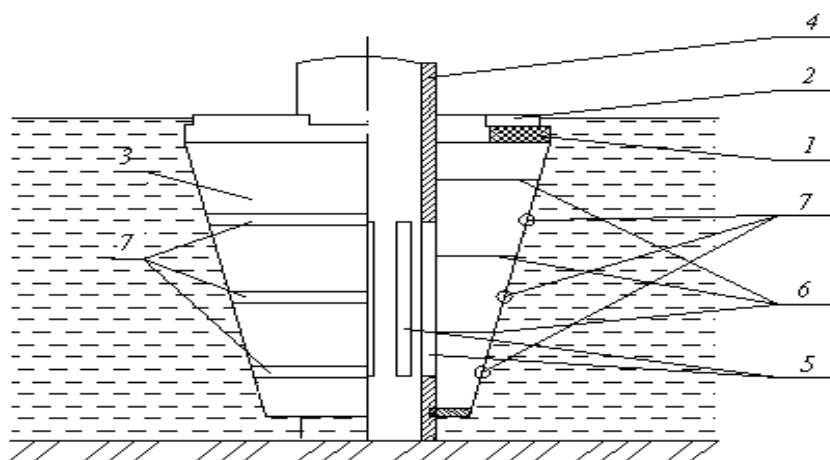
4 сурет – «Аманат» Орал техникалық институтында орындалған суды бетінен сорып алатын құрылғының конструктивтік –технологиялық сұлбасы
