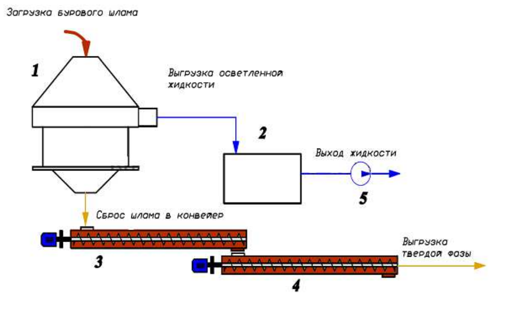
Рисунок 1 – Установка обезвреживания бурового шлама
