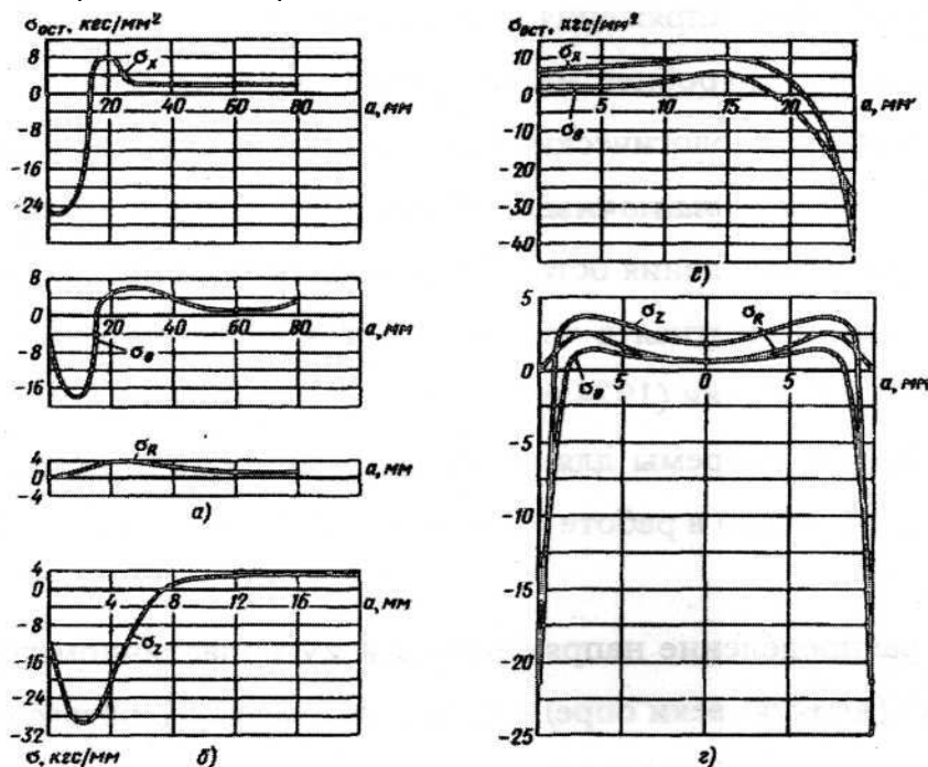
Рисунок 1 – Эпюры остаточных напряжений после обкатки роликами:
