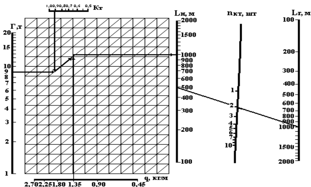
5 сурет – Танаптық кагаттардың санын және жинақталу арақашықтығын анықтауға арналған номограмма
