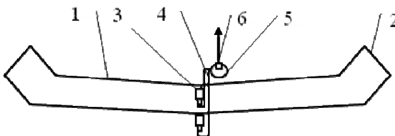
1 сурет – Екі қатарлы сиыр орнының сауын қондырғыларының сүтөткізгіштерінің біріктірілуі
