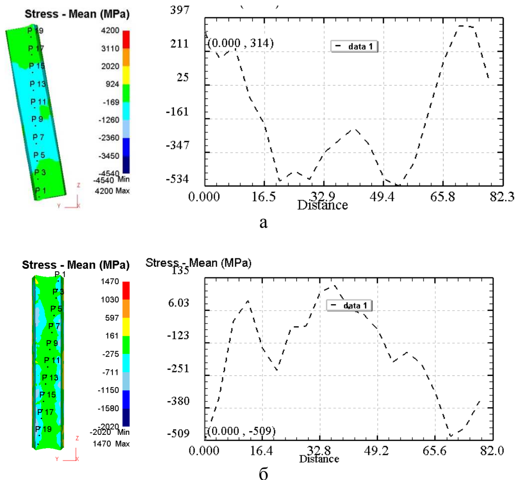
Рисунок 4 – Распределение средних напряжений по сечению полосы:
