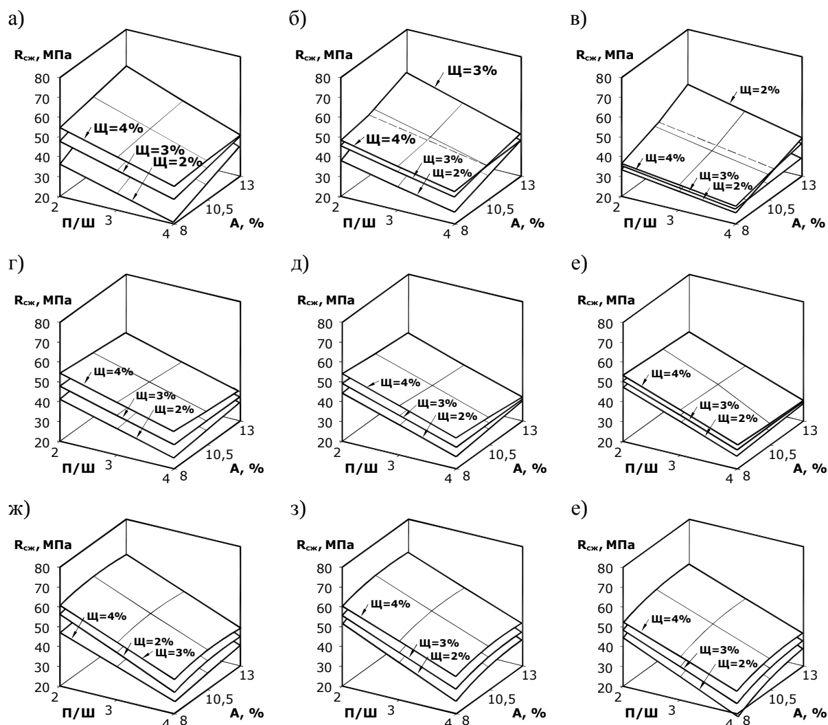
Рисунок 2 – Влияние состава минерально-щелочного вяжущего на прочность через 28 суток твердения в нормальных условиях (обозначения по рис. 1)
