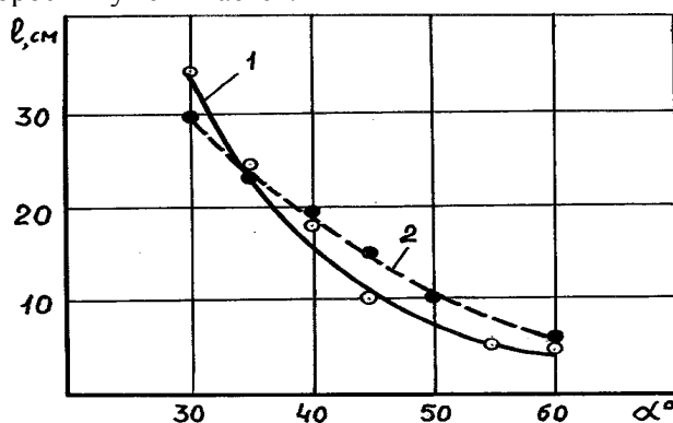
Рисунок 2 – Зависимость дальности полета отраженных зерен от угла падения при V = 4,3 м/с 1-пшеница; 2-ячмень
