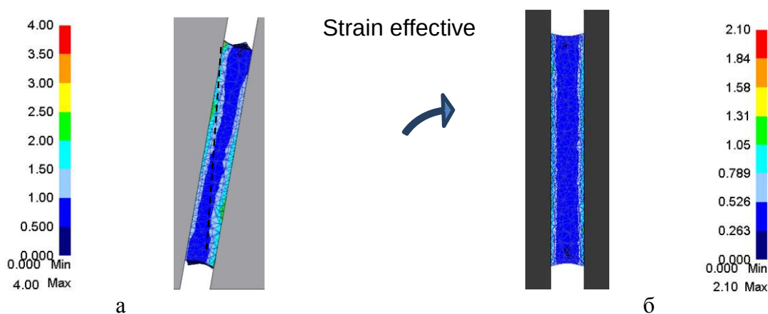
Рисунок 3 – Распределение эквивалентных деформаций по сечению полосы в процессе прокатки в валках с обратной конусностью; а – в валках с обратной конусностью; б – в цилиндрических валках
