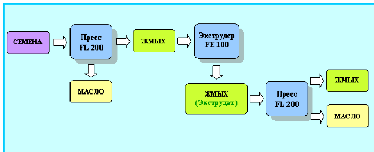
Рисунок 6 – Схема двукратного прессования с экструзией
