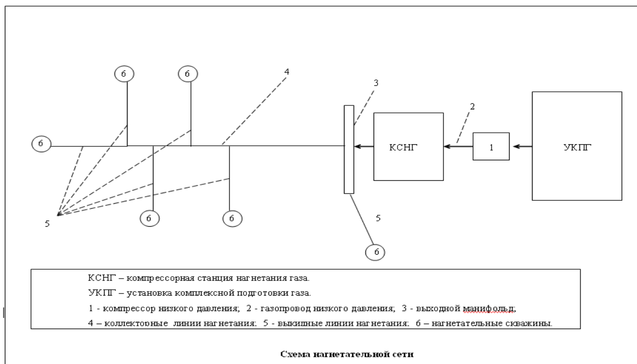
Рисунок 1 – Схема нагнетательной сети
