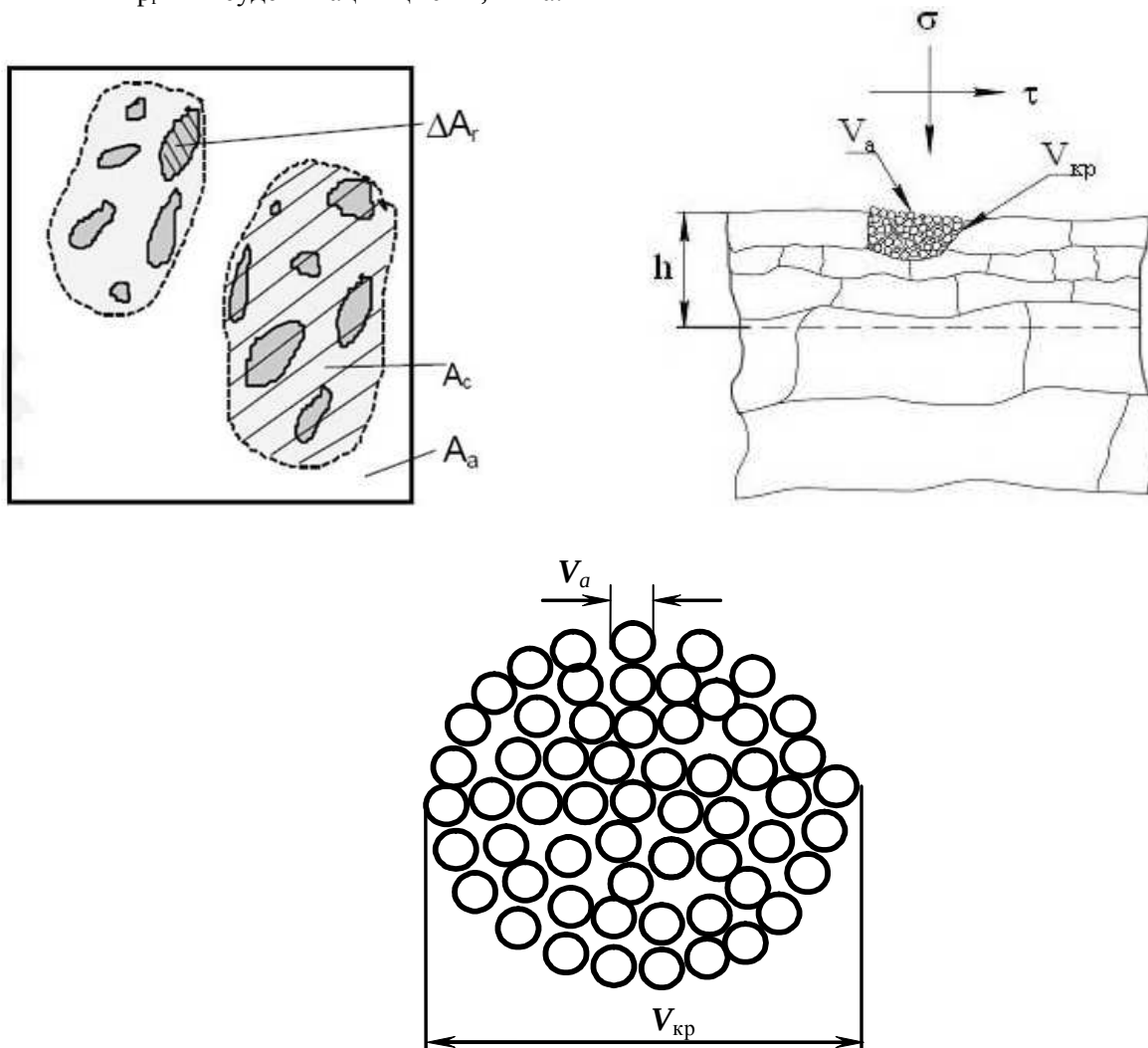
1 сурет – Тозық түйірінің қалыптасу сұлбасы: A_a – тиісудің номиналдық ауданы, мм 2 ; A_c – пішіндік аудан, мм 2 ; \Delta A_r – тиісу дағының бірлігінің нақты ауданы, мм 2 ; h – үйкеліс бетінің зақымдалуларының ең үлкен шоғырлануы орналасқан тереңдігі, мм; V_{kp} – орташа статистикалық тозық түйірінің көлемі, мм 3 ; V_a – элементарлы әрекеттелетін көлем, мм 3
