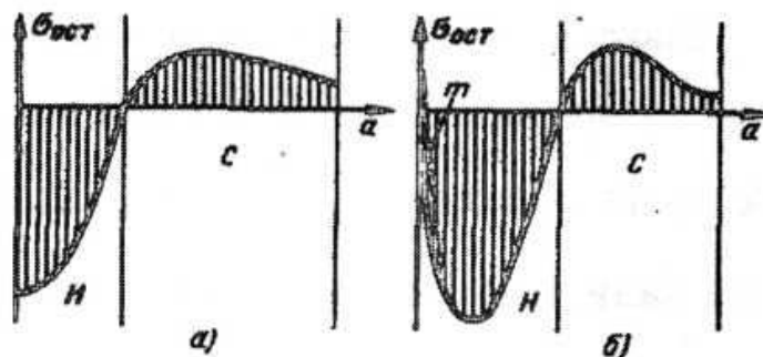
Рисунок 4 –Схема образования остаточных напряжений при неодновременных по сечению фазовых превращениях в процессе охлаждения
