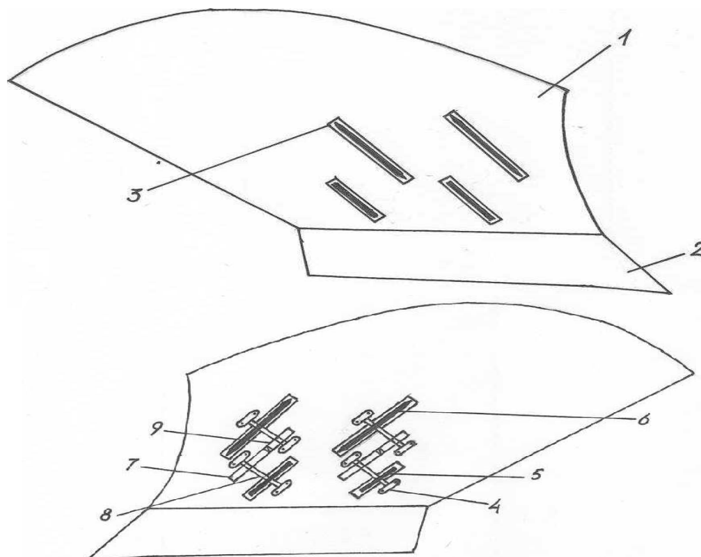
2 сурет – Соқа тұрқасын алдынан және артынан қарағандағы көрініс 1-қайырма, 2-түрен, 3-жырма, 4-подшипник, 7-бірінші деңгейдегі шестерня, 8-білік, 9-екінші деңгейдегі шестерня
