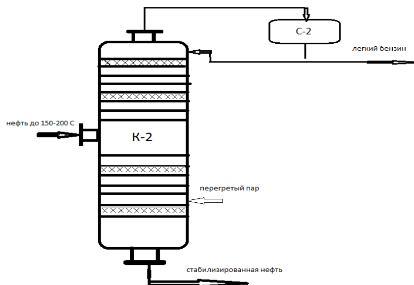
Рисунок 2 – Реконструкция отбензинивающей колонны
