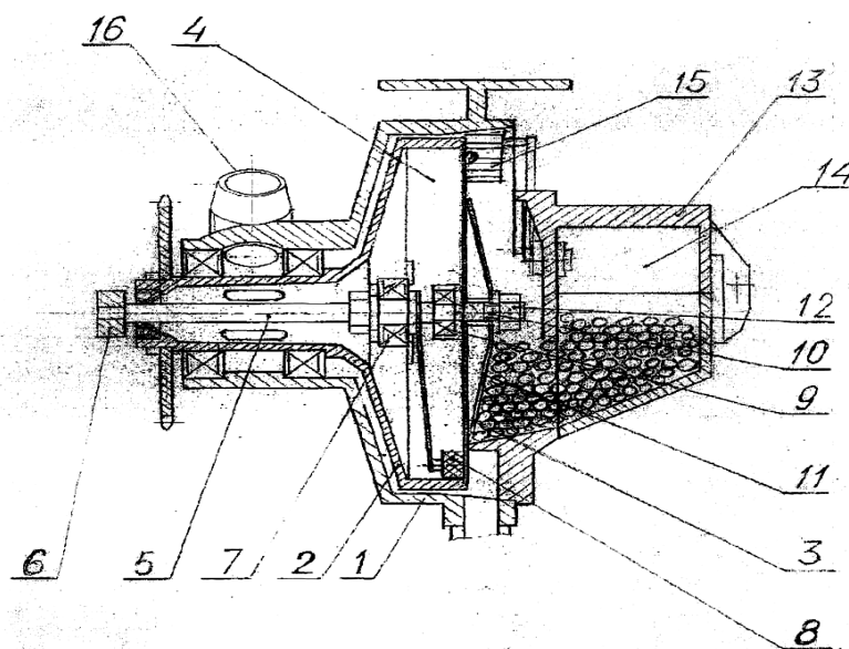
2 сурет – Пневматикалық тұқым себу аспабының құрылысы
