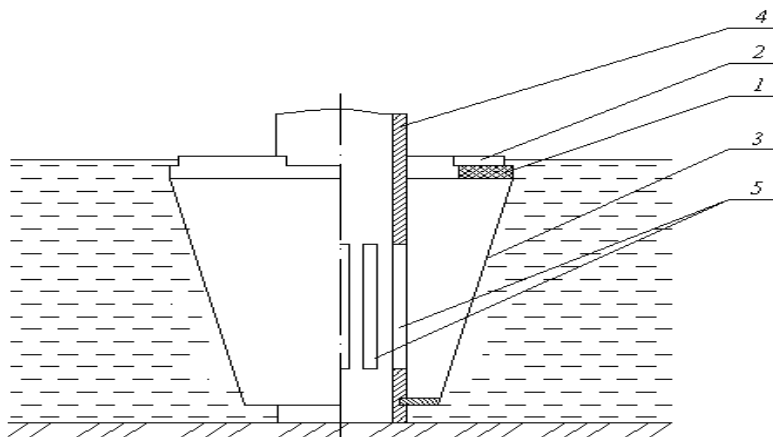
3 сурет – М. И.Калинин атындағы Түркімен ауыл шаруашылық институтында жасалған суды бетінен сорып алатын құрылғысының конструкциясының сұлбасы
