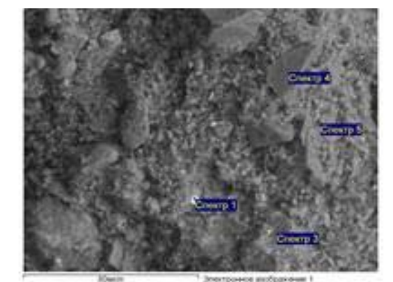
Рисунок 1 - Электронно-микроскопический снимок бентонитоподобной (монтмориллонитовой) глины Погадаевского месторождения Западно-Казахстанской области
