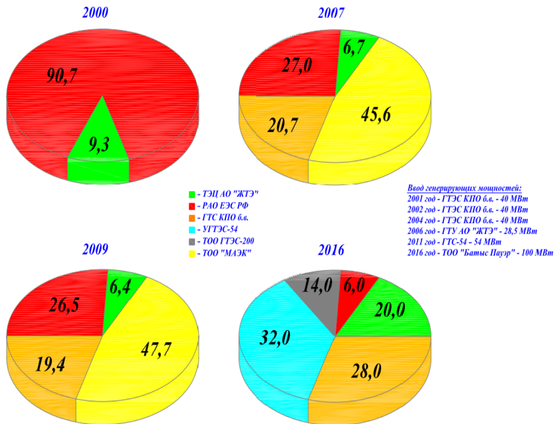
Рисунок 1 - Структура поставок электроэнергии по АО «Зап.-Каз.РЭК»
