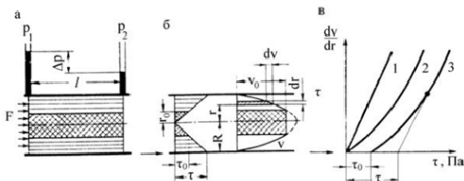
Рисунок - 1. Движение ньютоновских и неньютоновских жидкостей по трубам: а – модель течения жидкости; б – распределение напряжений и скоростей в структурном потоке; в – зависимость напряжений сдвига от градиента скорости для ньютоновских 1 и неньютоновских 2, 3 жидкостей
