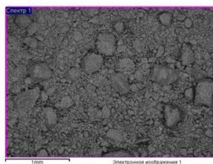
Рисунок 2 - Химический элементный состав, микроструктура и спектр кремнистой породы – опоки Таскалинского месторождения
