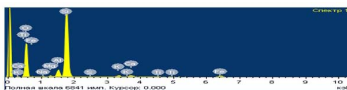
Рисунок 2 - Химический элементный состав, микроструктура и спектр кремнистой породы – опоки Таскалинского месторождения
