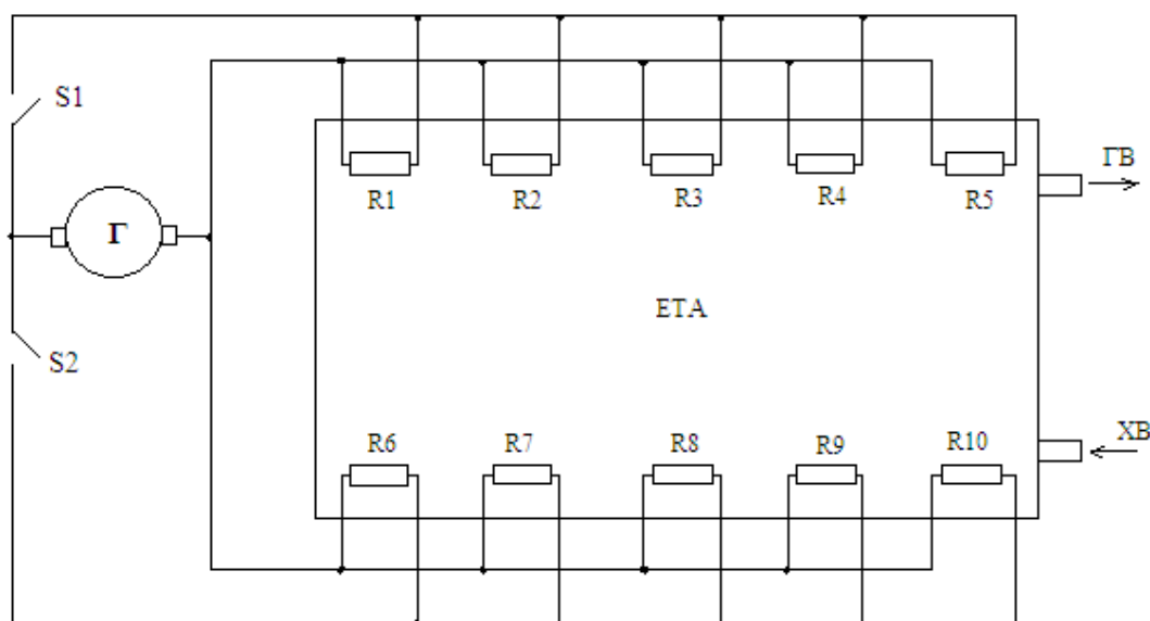
Рисунок 2 - Электрическая схема подключения нагревателей к ветрогенератору:
