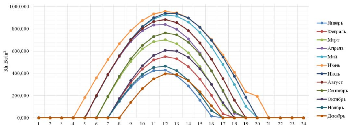
Рисунок 2 - Мощность потока солнечной радиации за каждый 15-й день каждого месяца
