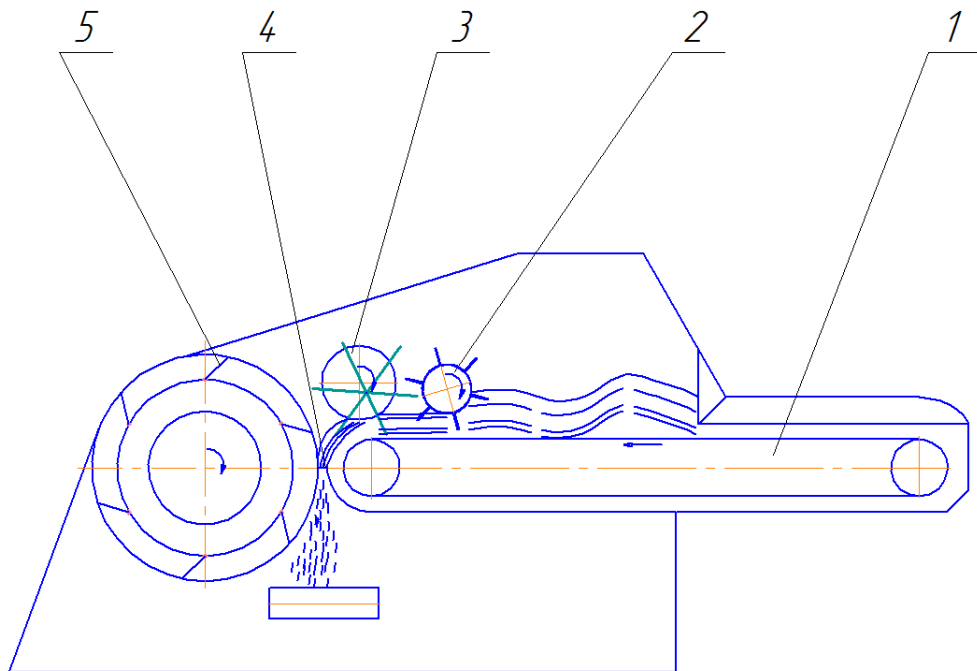
1-подающий транспортер, 2-ваlec с гребенками, 3-прочесывающий битер, 4-противорежущая пластина, 5-измельчающий аппарат
