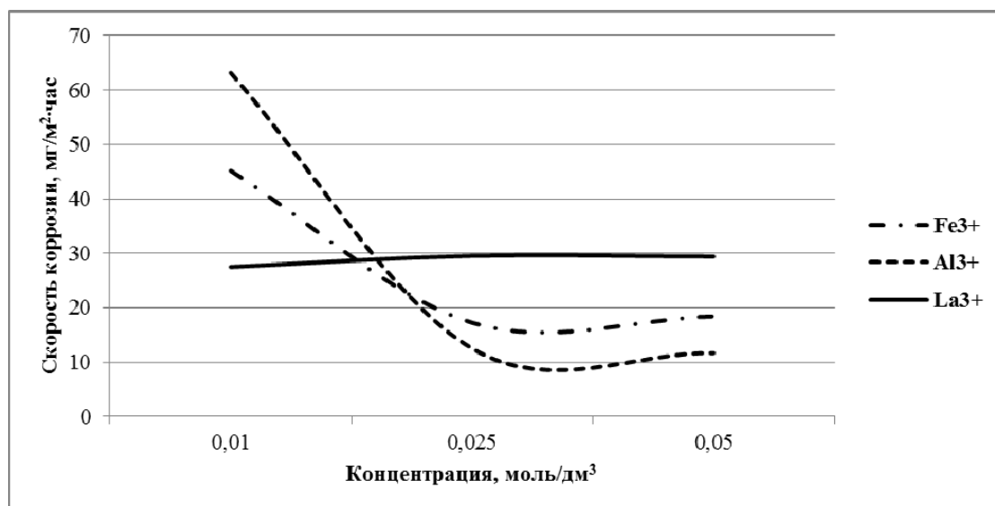
Рисунок 1 – Зависимость скорости коррозии стали Ст-3 от концентрации гидрофосфата натрия в присутствии ионов-модификаторов
