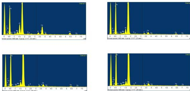
Рисунок 2 - Спектры исследуемых участков бентонитоподобной (монтмориллонитовой) глины
